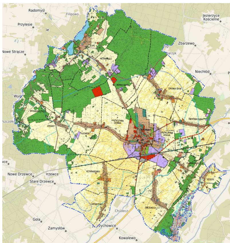
Ryc. 1. Studium uwarunkowań i kierunków zagospodarowania przestrzennego Gminy Wschowa
